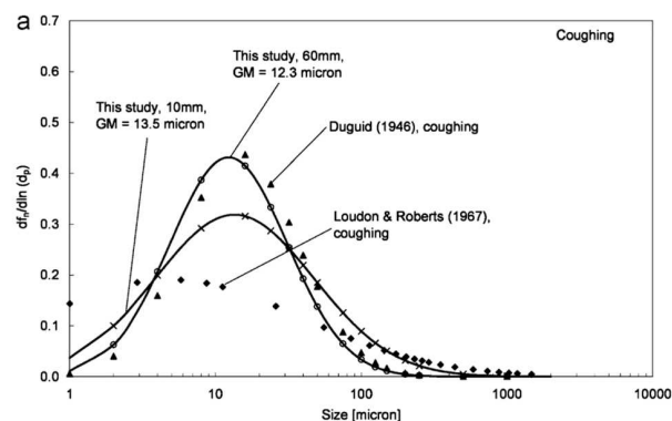
人から排出される飛沫の大きさと割合 10 \mu\text{m} 程度の大きな飛沫が多い Chao et al., Aerosol Science 40(2009)122-133)
