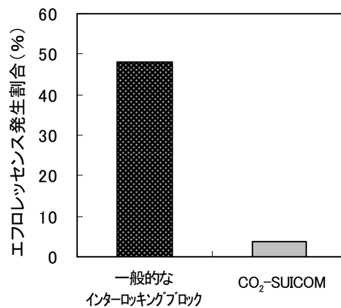
図 6 エフロレッセンスの発生割合
