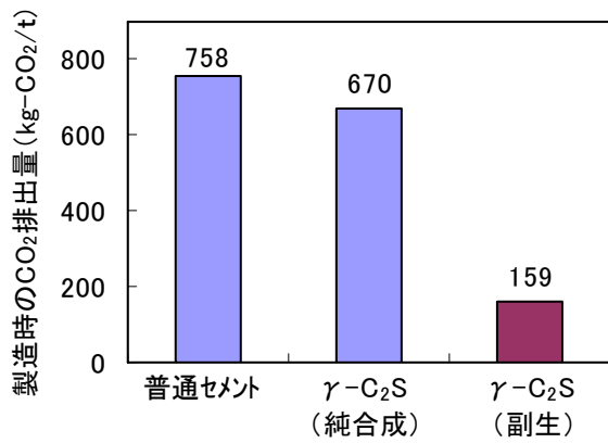
図3 γ-C 2 SのCO 2 排出量
