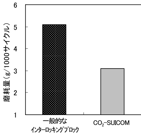
図 5 CO 2 -SUICOM の耐摩耗性
