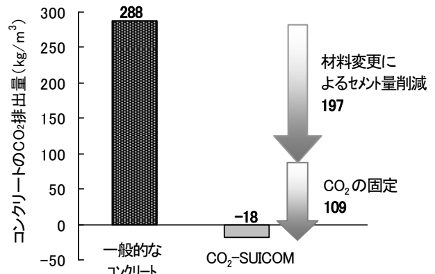
図4 コンクリートのCO 2 排出量
