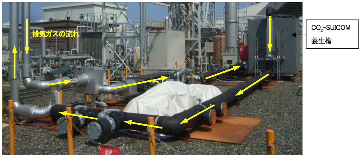
写真1 炭酸化養生設備
