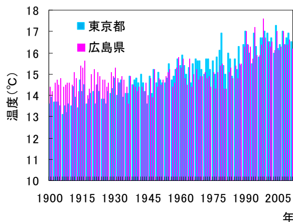
図 1 東京都と広島県の平均気温の変化 (気象庁のデータをもとに作図)
